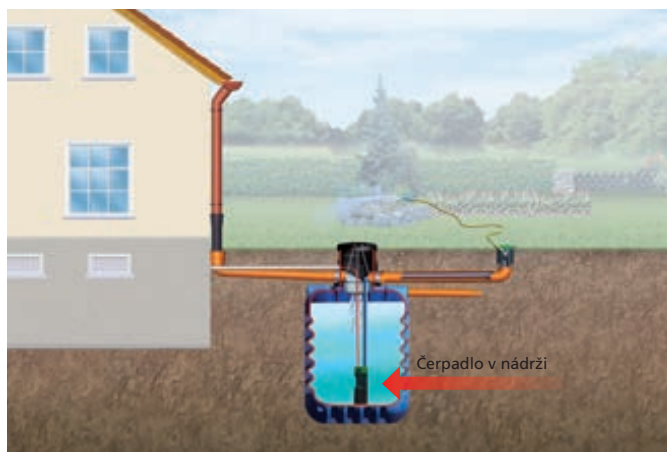
Sada na čerpanie – Garden Comfort 504,00 Typ: 7962
